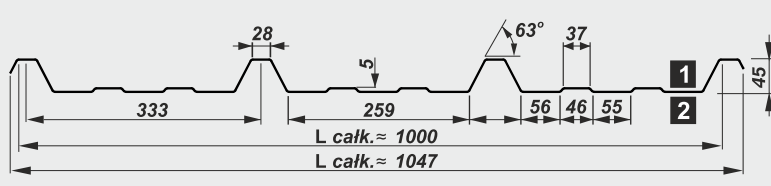
PROFIL DACHOWY
