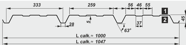
PROFIL ELEWACYJNY
